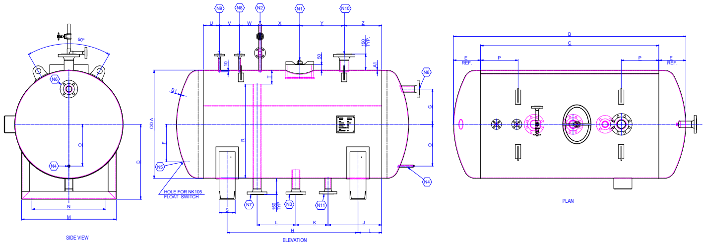
DIMENSIONEN
